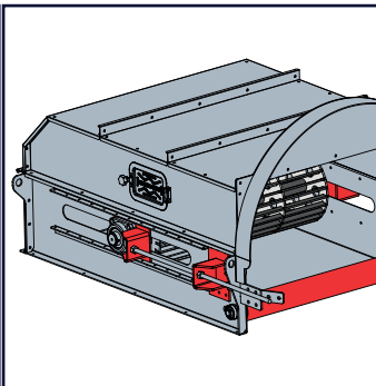
Gerdirme Mekanizması
