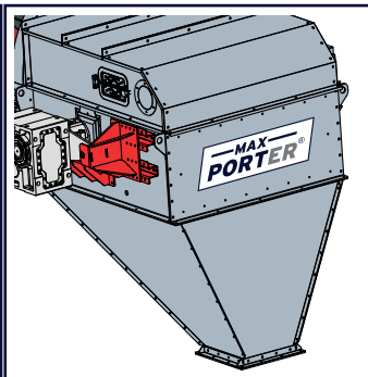
Döküş Haznesi
